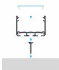
Manual de instalação do perfil ILEDO com tampa WIDE, com parafuso de fixação
